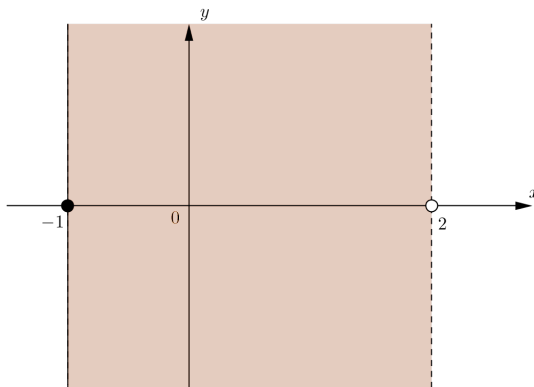
Figura 3.1: Região do conjunto solução da inequação em \mathbb{R}^2 .
