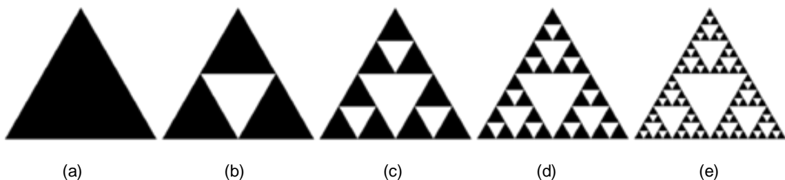
Figura 21: Triângulo de Sierpinski
