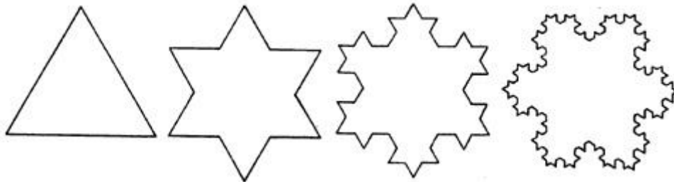
Figura 22: Curva de Koch
