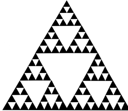
Figura 20: Triângulo de Sierpinski
