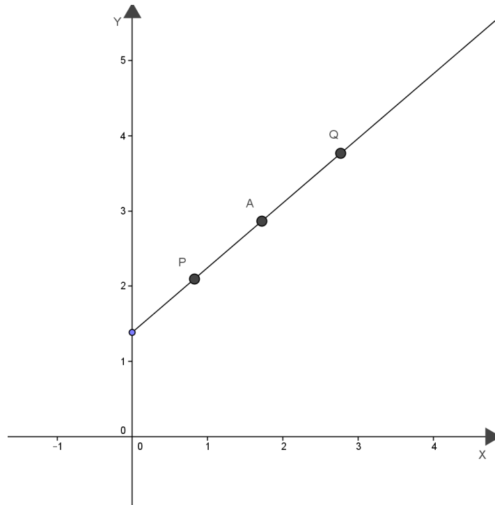
Figura 10: Gráfico de uma função afim.
