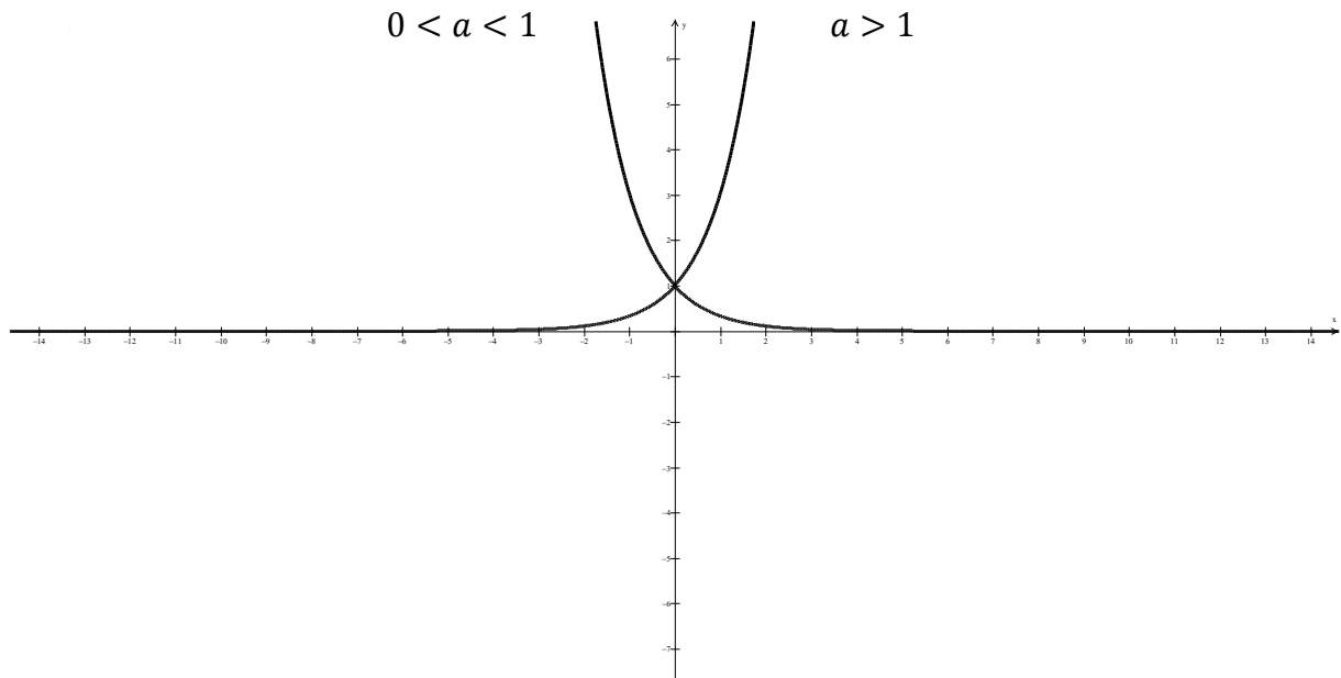
Figura 15 Gráfico da função exponencial
