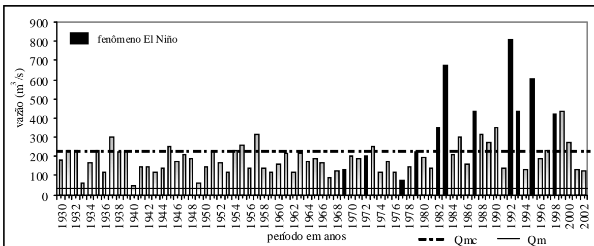
Gráfico 18 - Vazões máximas anuais, seção Rio dos Patos – período 1930 - 2002
